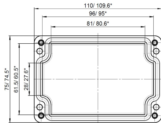
Deckel / lid
